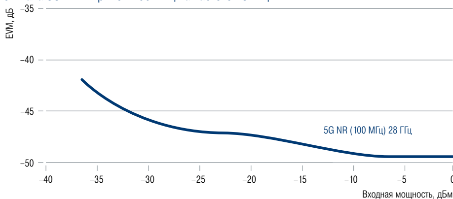
Остаточный EVM в зависимости от мощности сигнала для восходящего сигнала 5G NR шириной 100 МГц на частоте 28 ГГц
